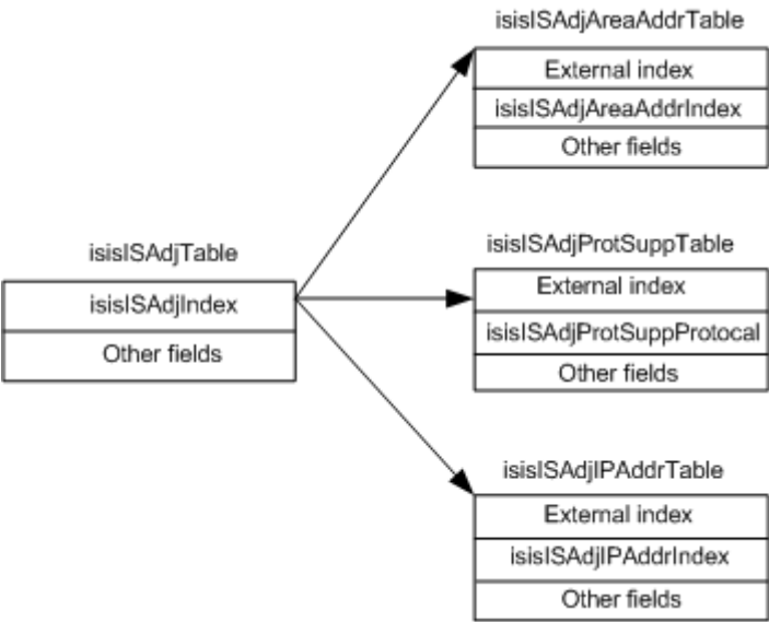
图 151-3 ISAdj 的表间关系图
